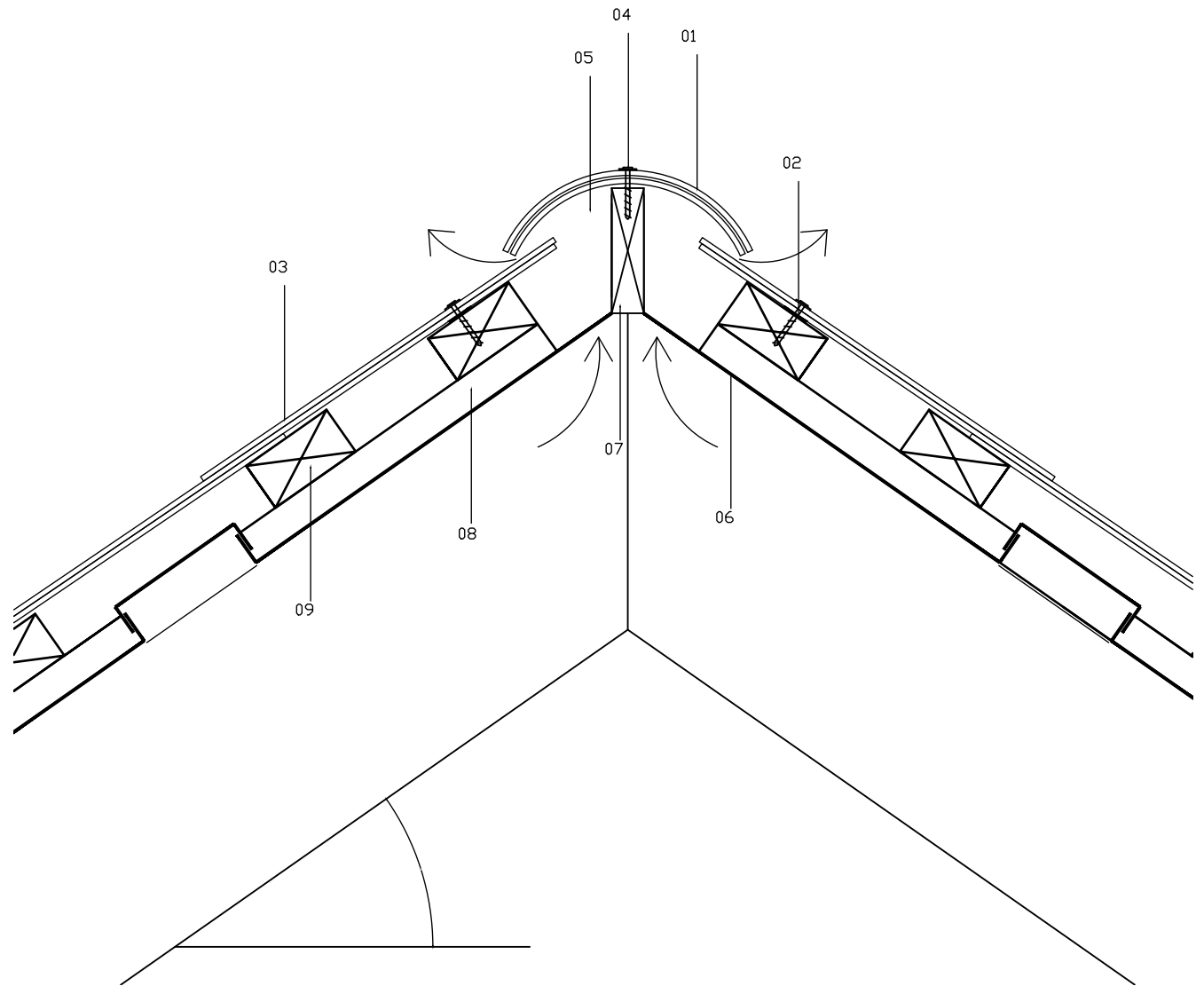
Loddrett snitt - Innvendig møne med konisk møne
